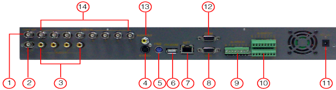
8-channel DVR 背板說明
