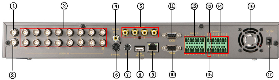
16-channel DVR 背板說明
